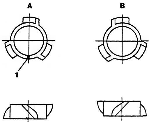
Fig. 62 Impeller
